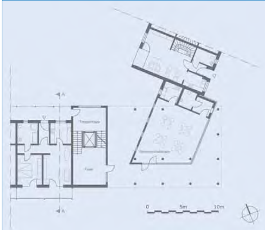
Grundriss des Eingangsbereichs mit Servicebüro und Gemeinschafts- raum.
