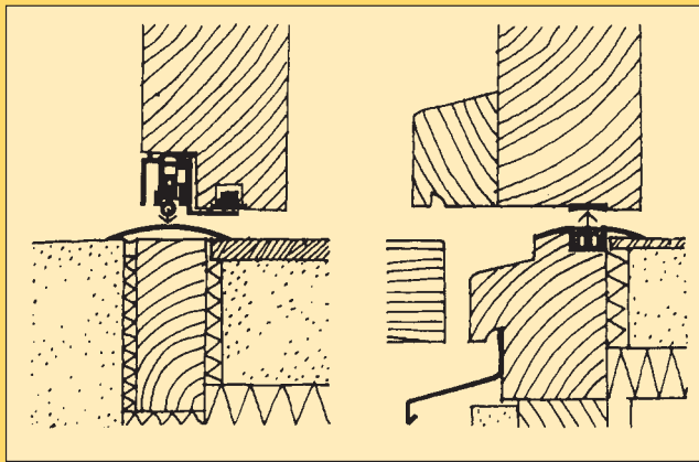
Dichtungen für Außentüren. Links: Hebedichtung, rechts Magnetdichtung. (Nach: Bayrisches Staatsministerium des Innern (Hg.), Wohnen ohne Barrieren, 1995.)
